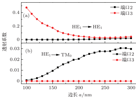
图6 (网刊彩色) HE_1 模式 SPPs 透射系数 (a) HE_1 输出; (b) TM_0 输出
